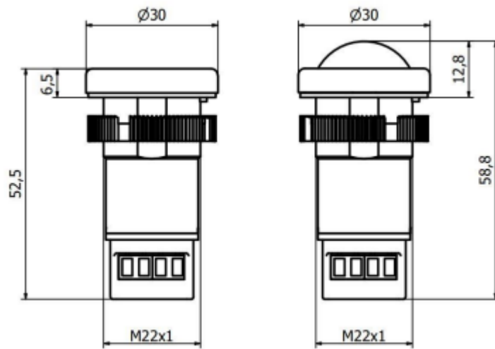
MD22DUO P
